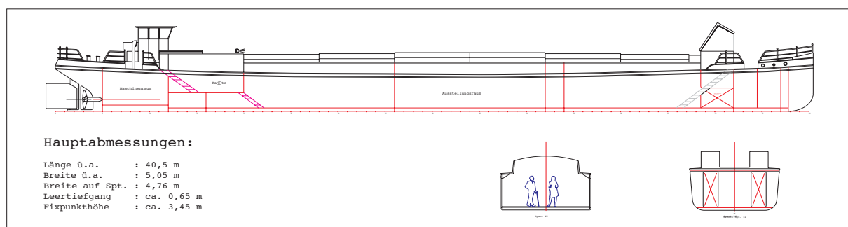
EDELWEISS (Finowmaßkahn), Baujahr 1930, Stahl, 296 BRT
